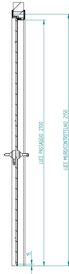
SEZIONE A-A
