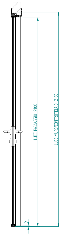
SEZIONE A-A
