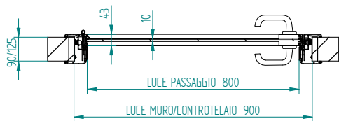
SEZIONE B-B
