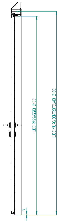
SEZIONE A-A
