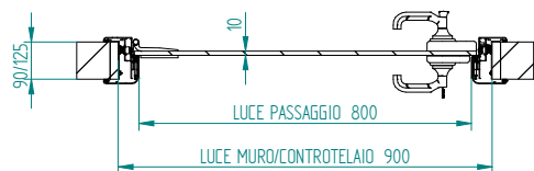
SEZIONE B-B
