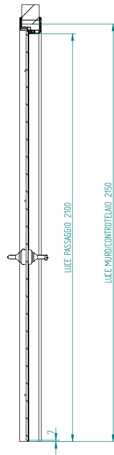
SEZIONE A-A
