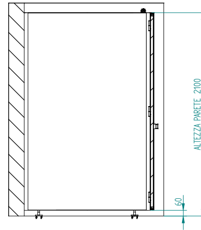
SEZIONE A-A
