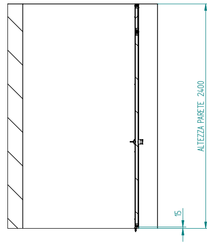
SEZIONE B-B
