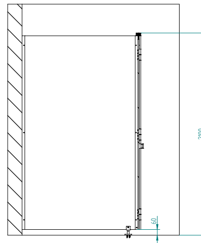
SEZIONE B-B
