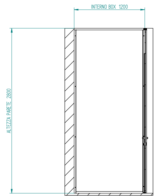
SEZIONE A-A
