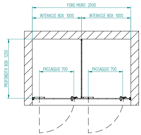
SEZIONE B-B
