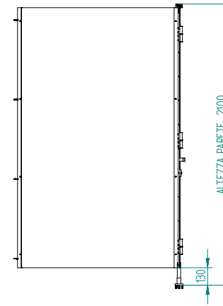
SEZIONE A-A
