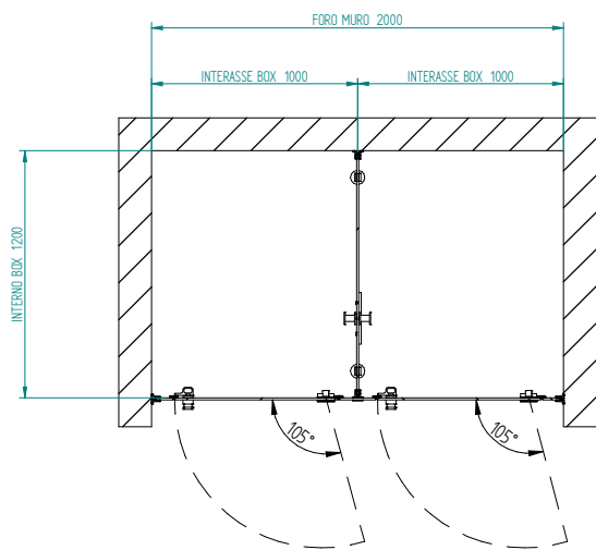
SEZIONE A-A
