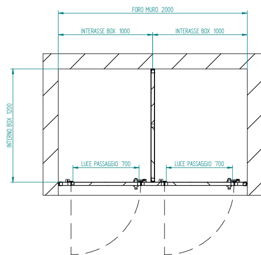
SEZIONE B-B
