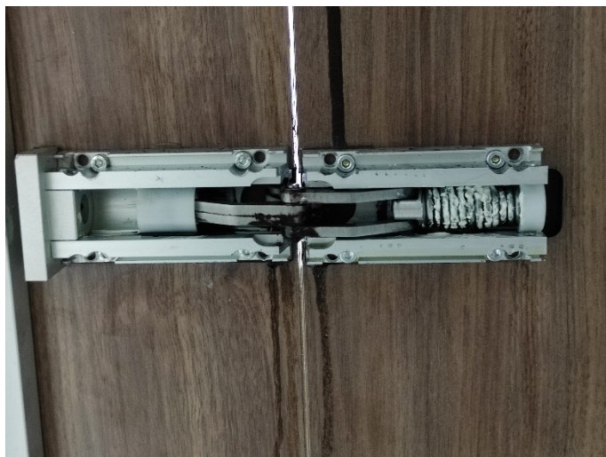
Fotografie della cerniera centrale al termine della prova in posizione di apertura e di chiusura
